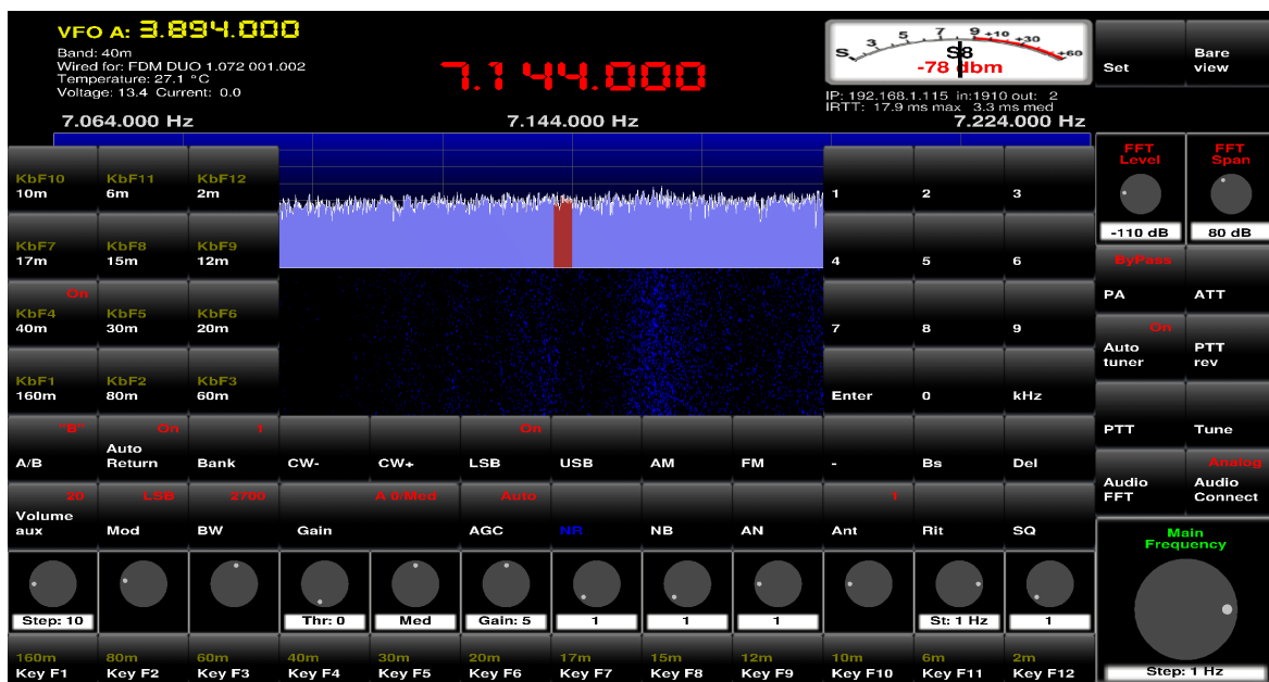
Schermata di impostazione bande, modi, frequenze
